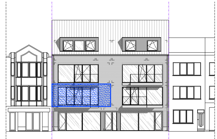
Vorgevel
