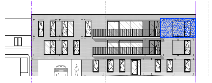
Vorgevel
